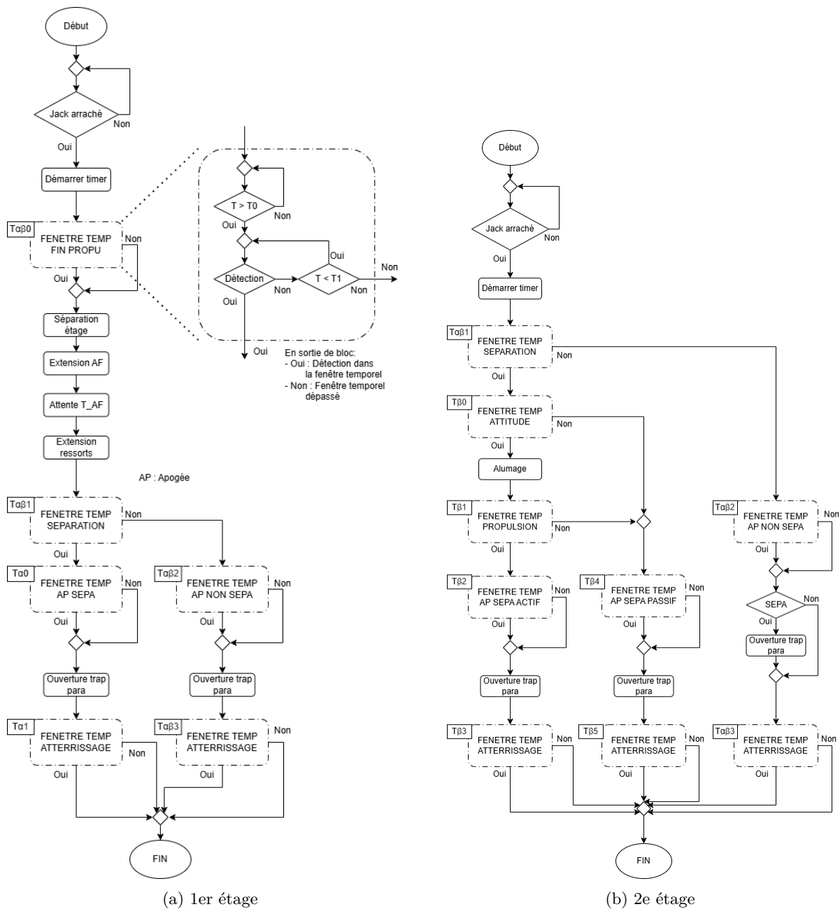
FIGURE 6.1 – Schémas fonctionnels des séquenceurs des deux étages
