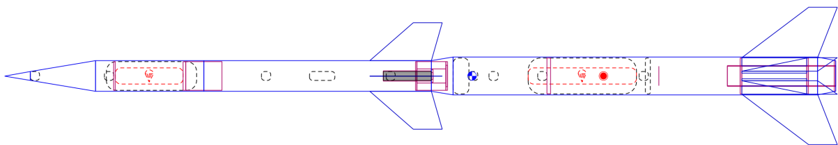
FIGURE 2.2 – Modélisation de la fusée SP-02 dans OpenRocket
